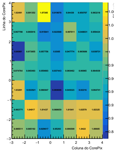
\epsilon_1^1(\text{CP0}): \text{Jan24-Mar6}
