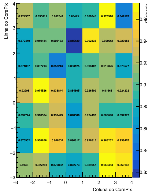
\epsilon_3^1(\text{CP0}): \text{Jan24-Mar6}
