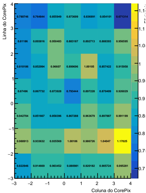
\epsilon_1^1(\text{CP0}) : Jan14-Feb23
