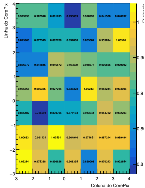
\epsilon_3^3(\text{CP0}) : Jan14-Feb23
