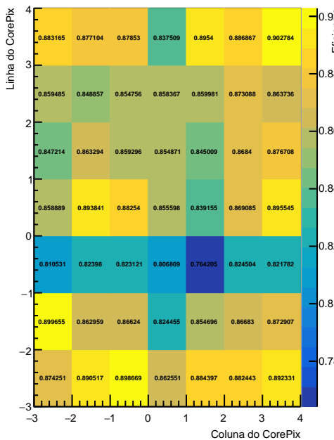
\epsilon_2^3(\text{CP0}) : Jan14-Feb23
